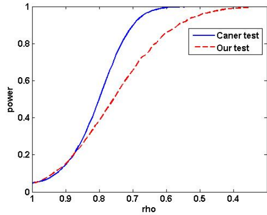
(d) \alpha = 1.9, T = 100
