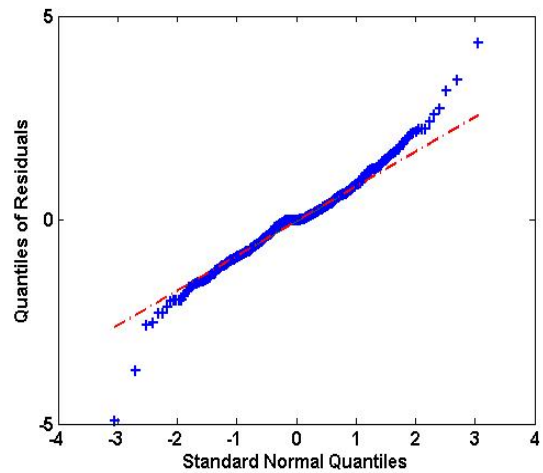
(d) U.K. residuals from VAR(12) ( \alpha = 1.85 )
