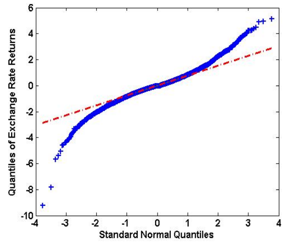
(d) U.K. residuals
